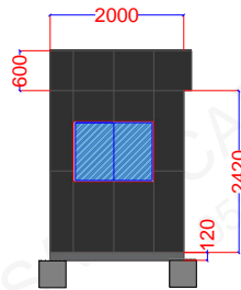
RIGHT ELEVATION
